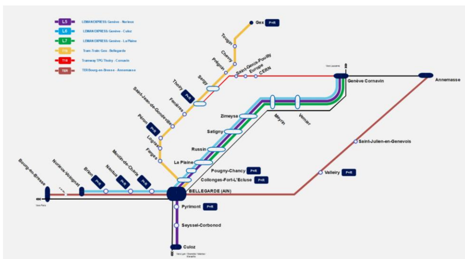
© Alain Teddy Mayaud, Schéma de l'Etoile de Bellegarde
